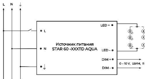
Рисунок 2 – Схема подключения
