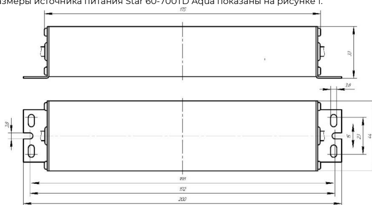
Рисунок 1 – Габаритные размеры Star 60-700TD Aqua
